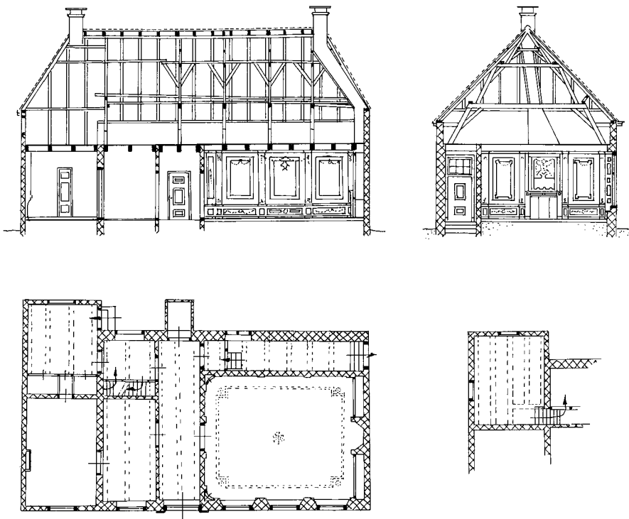
Toestand voor de restauratie naar een opmeting uit 1977: voor- en achtergevel, west- en oostgevel, langs- en dwarsdoorsnede, plattegrond begane grond en kelder.
