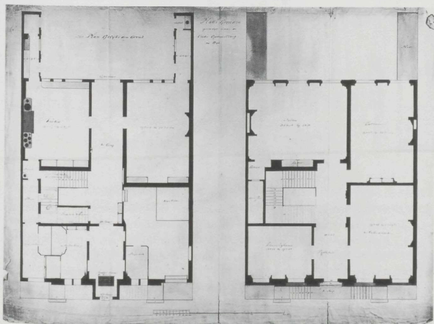
Toestand 18de eeuw. Opmeting uit 1792, mogelijk door B.W.H. Ziesenis. Bij de restauratie van 1940 onder leiding van C.W. Royaards kreeg het huis opnieuw deze indeling.
