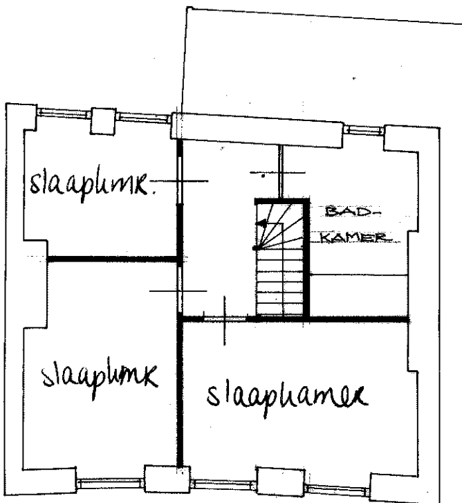
1E VERDIEPING
