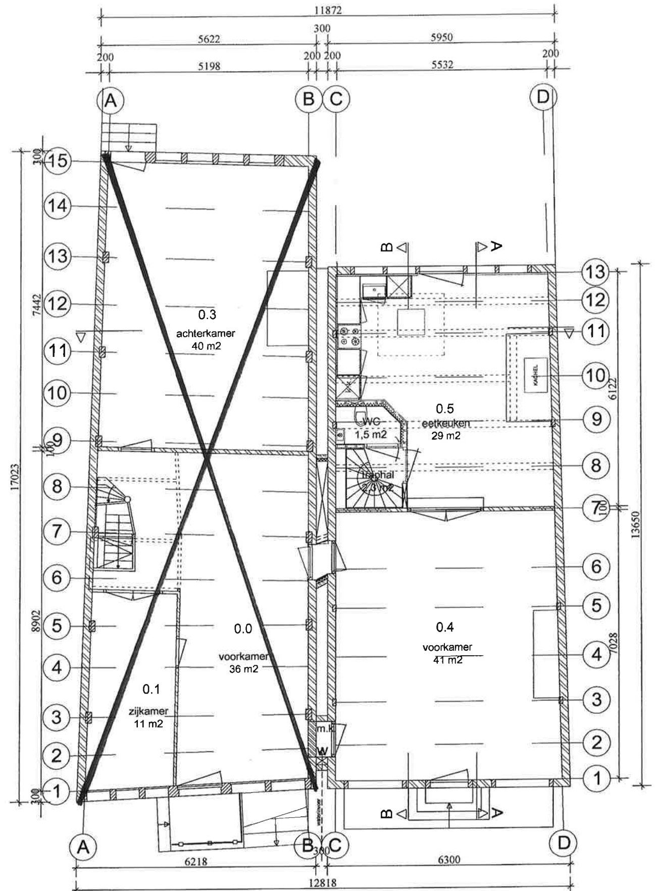
Begane grond Binnenluidendijk 4
