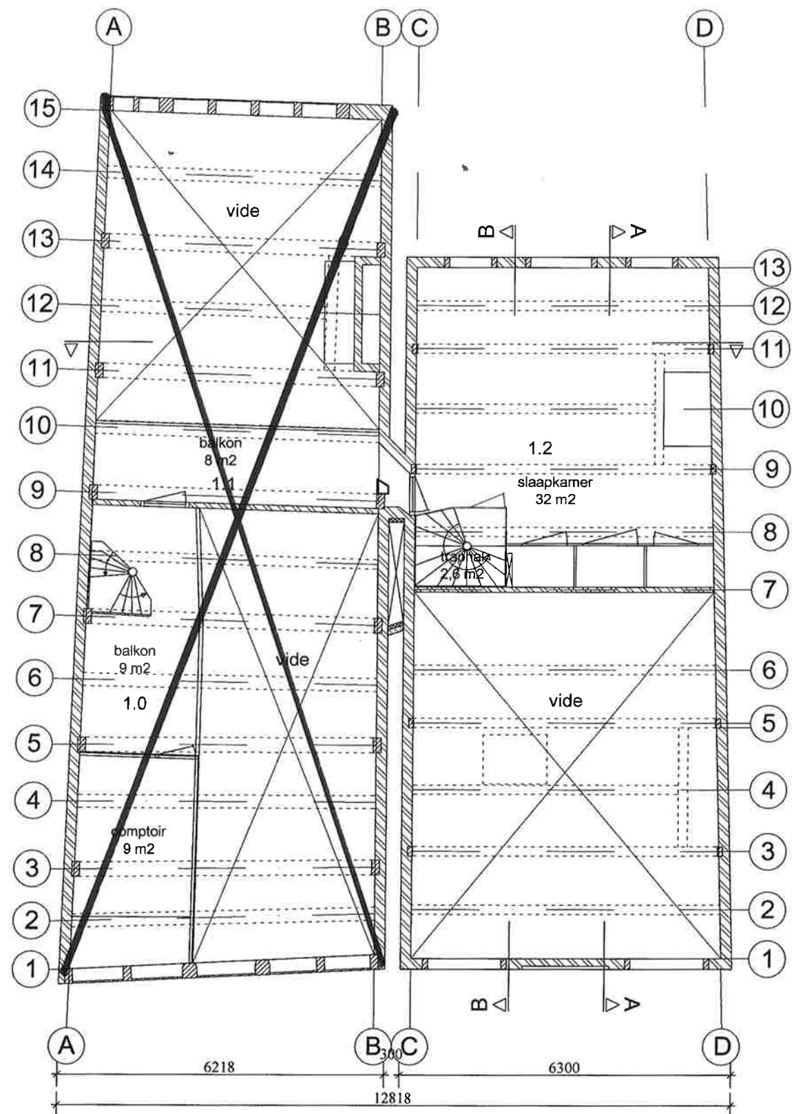
1e verdieping Binnenluidendijk 3
