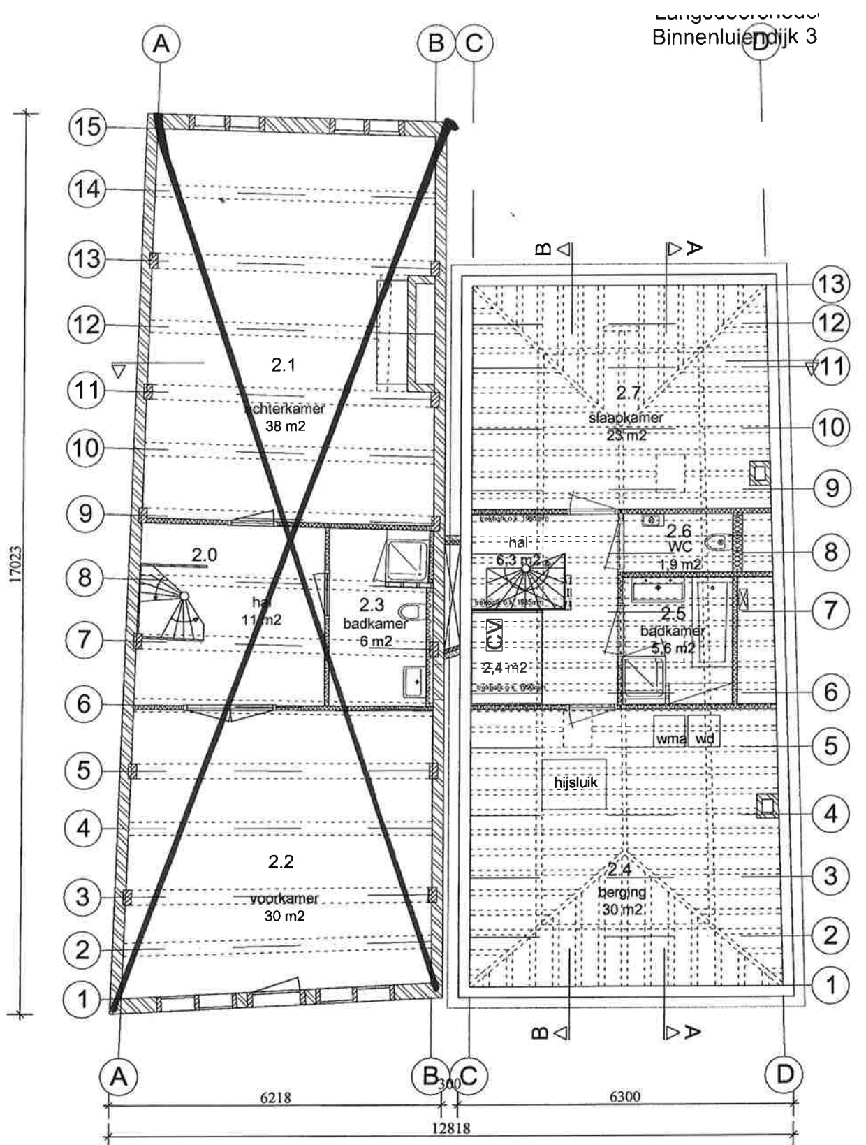
2e verdieping Binnenluidendijk 3
