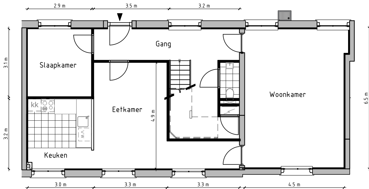
Lindenhof 8 (binnenouderswoning) | Begane grond 1:100
