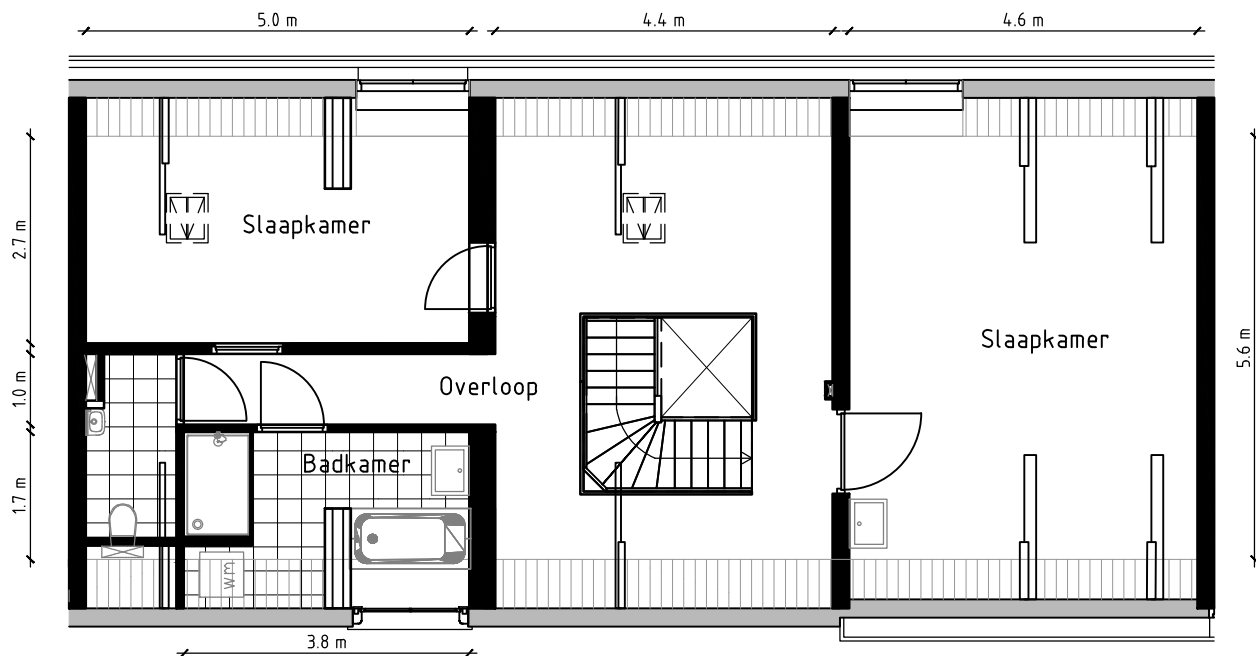
Lindenhof 8 (binnenouderswoning) | Verdieping 1:100
